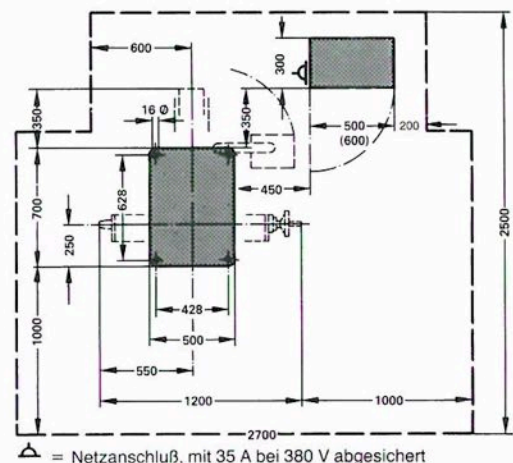
Fundamentplan und Platzbedarf mit Sicherheitsbereich
